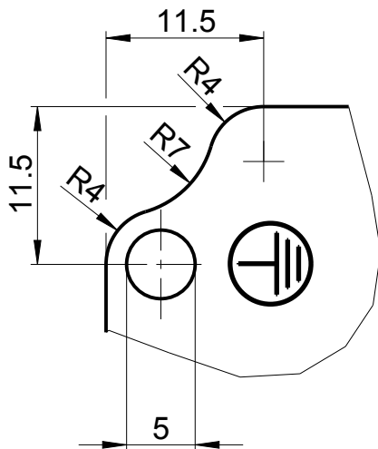
Einzelheit "X" 2:1
