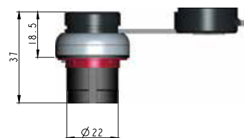
Måltegnig
