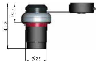
Måltegnig
