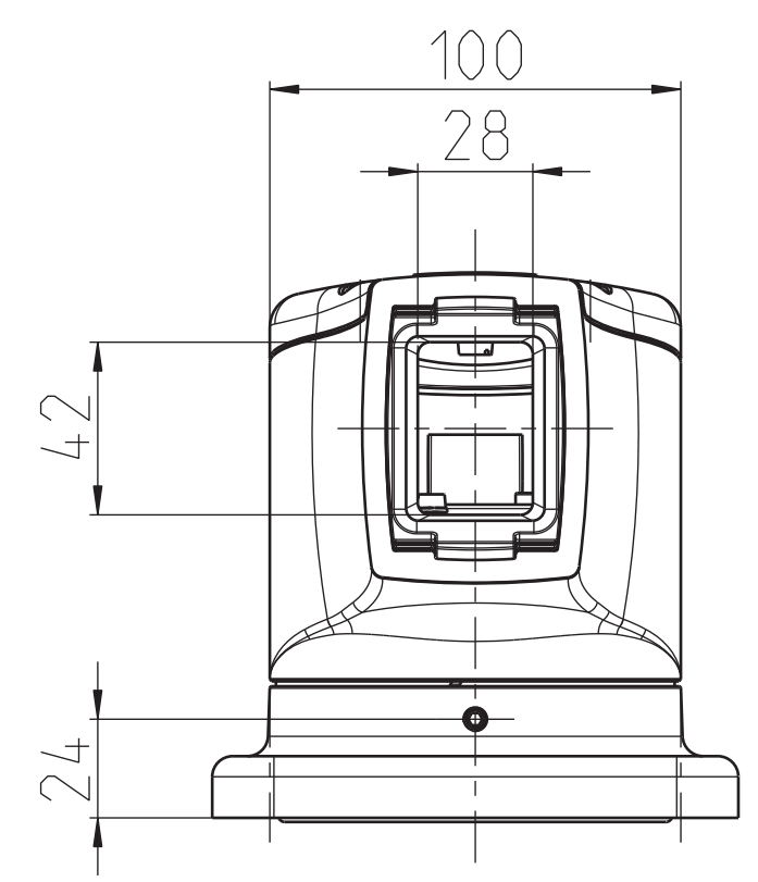
Bearbeitungszeichnung für Montagefläche
