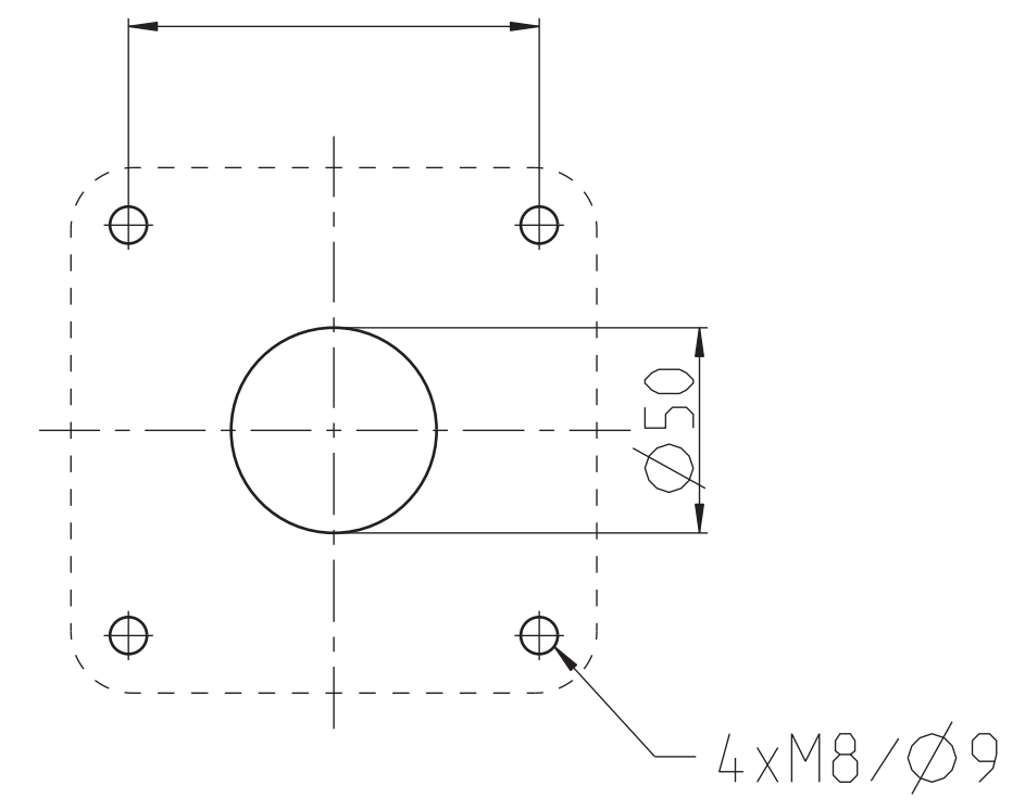
Bearbeitungszeichnung für Montagefläche
