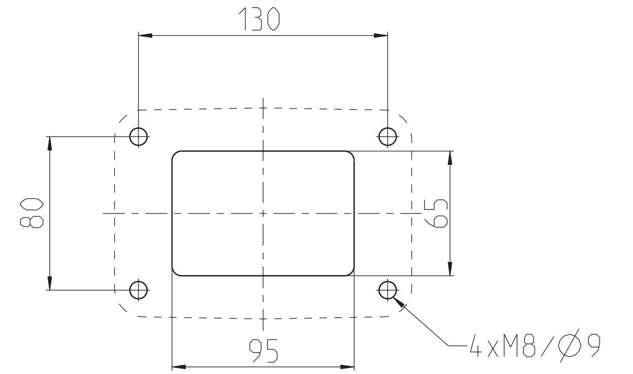
Bearbeitungszeichnung für Montagefläche
